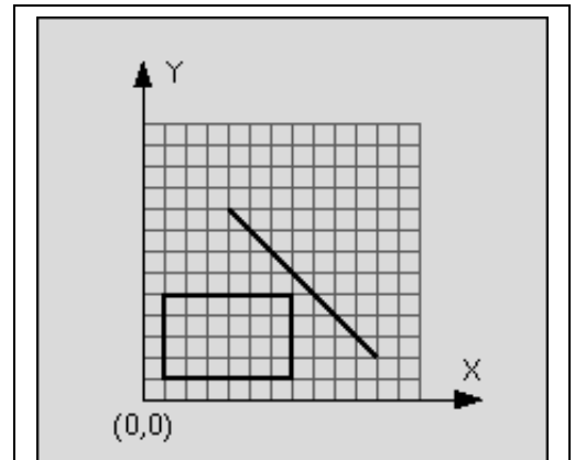
Εικόνα 23 Γραμμή δεν τέμνει ορθογώνιο
