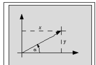
Εικόνα 24 Η γωνία κλίσης ενός διανύσματος
